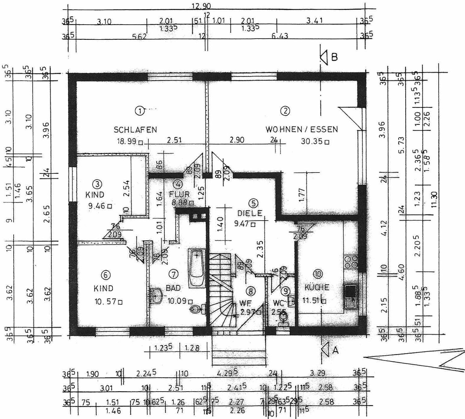
ERDGESCHOSS
