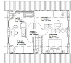
Grundriss DG
