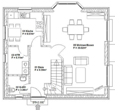
Grundriss EG
